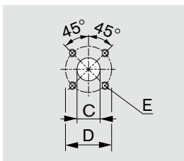
20 矩形法兰
